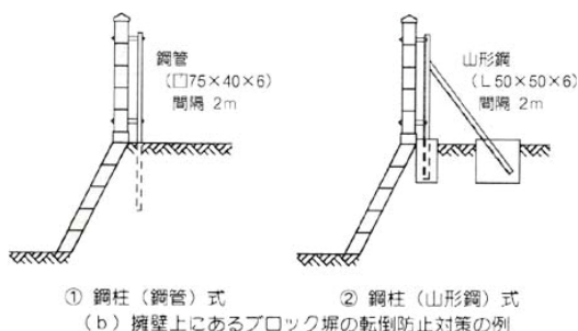
(b) 擁壁上にあるブロック塀の転倒防止対策の例
