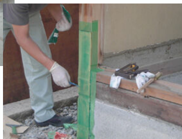
柱脚補強 (70cmシート1枚貼り)
