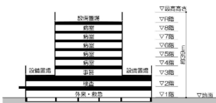
西-東 断面図
